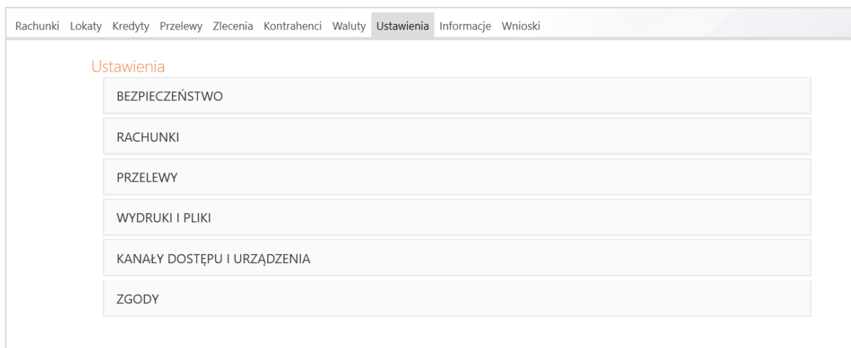
Rys. 43 Okno „Ustawienia”
